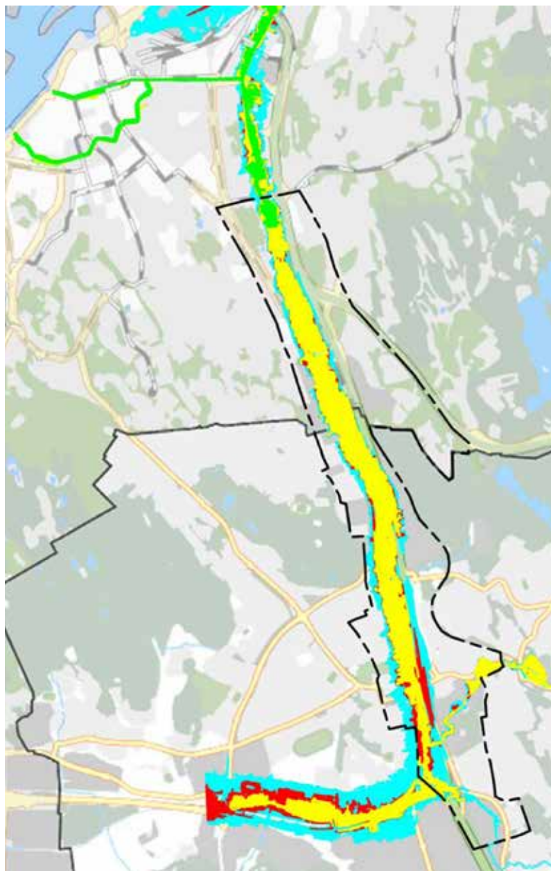
Översvämningskartering
